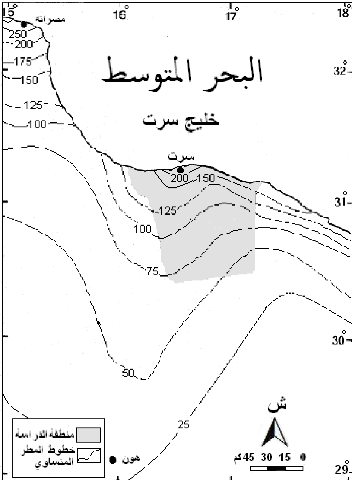
شكل رقم (22) خطوط المطر المتساوي بمنطقة الدراسة وما جاورها
