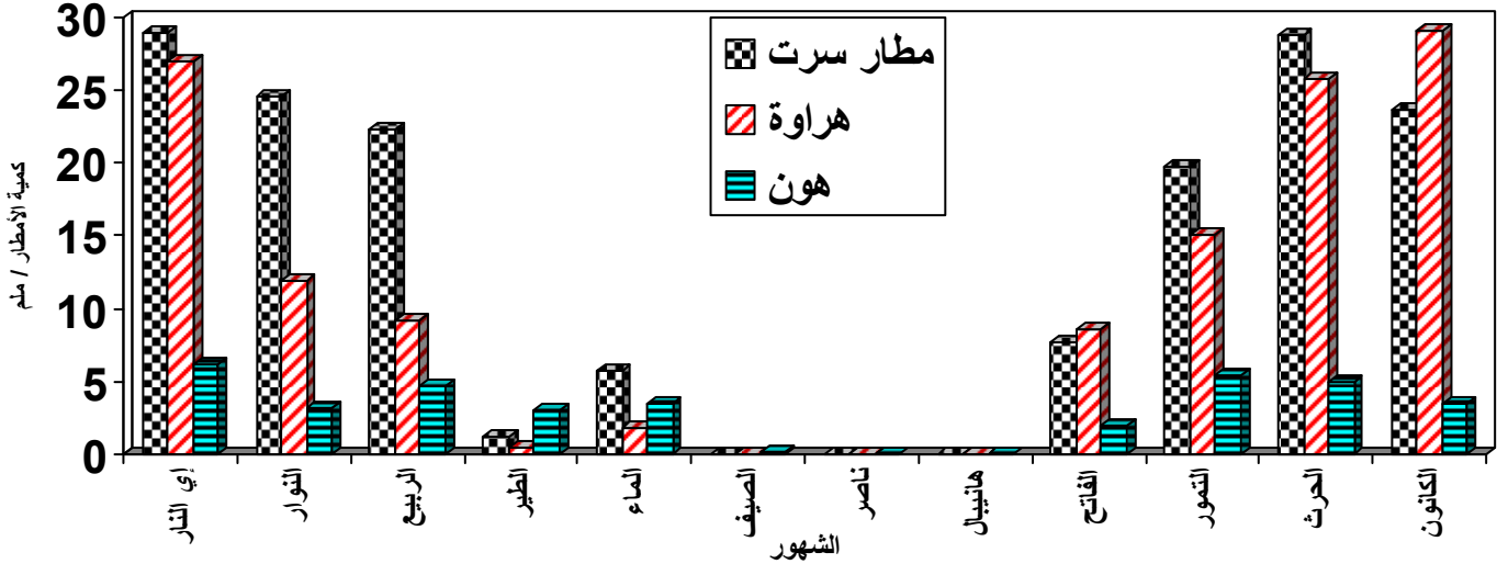
شكل رقم ( 21 ) التوزيع الشهري للأمطار بمحطات مطار سرت ، هراوة ، هون .
