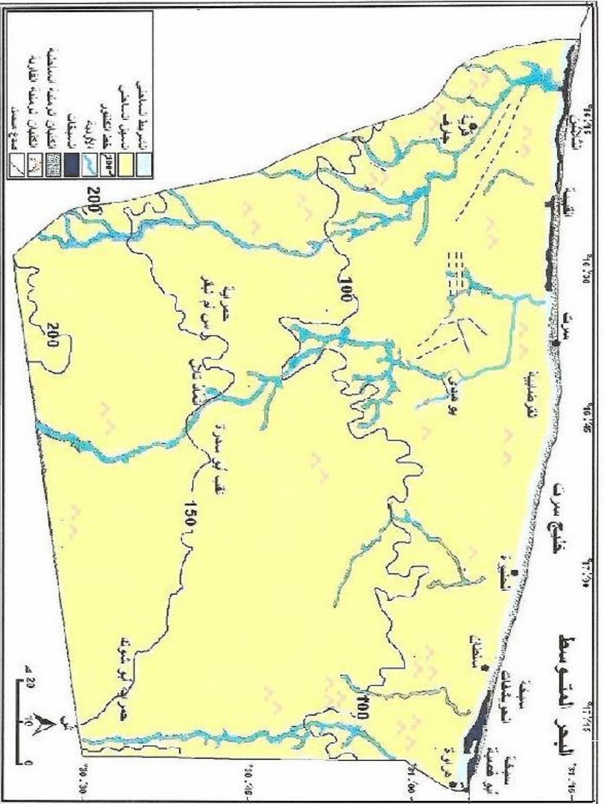
شكل رقم (4) جيو مورفولوجية منطقة اندر اسنة
