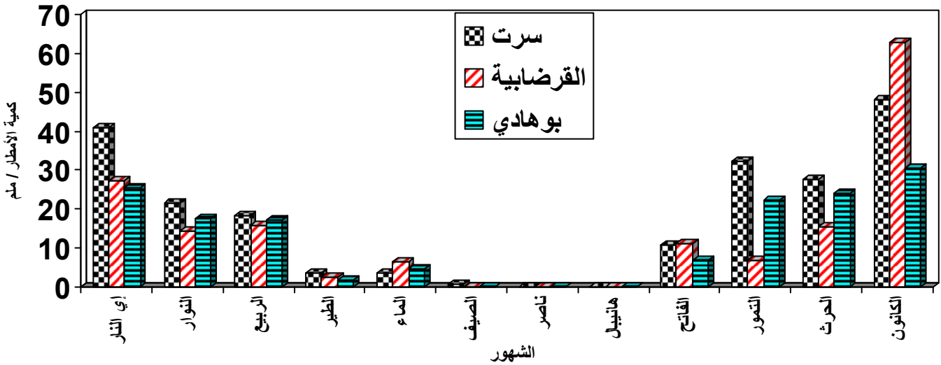
شكل رقم ( 20 ) التوزيع الشهري للأمطار بمحطات سرت ، القرصابية ، بوهادي .
