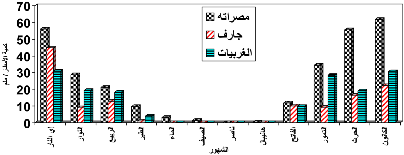
شكل رقم ( 19 ) التوزيع الشهري للأمطار بمحطات مصراته ، جارف ، الغربيات .
