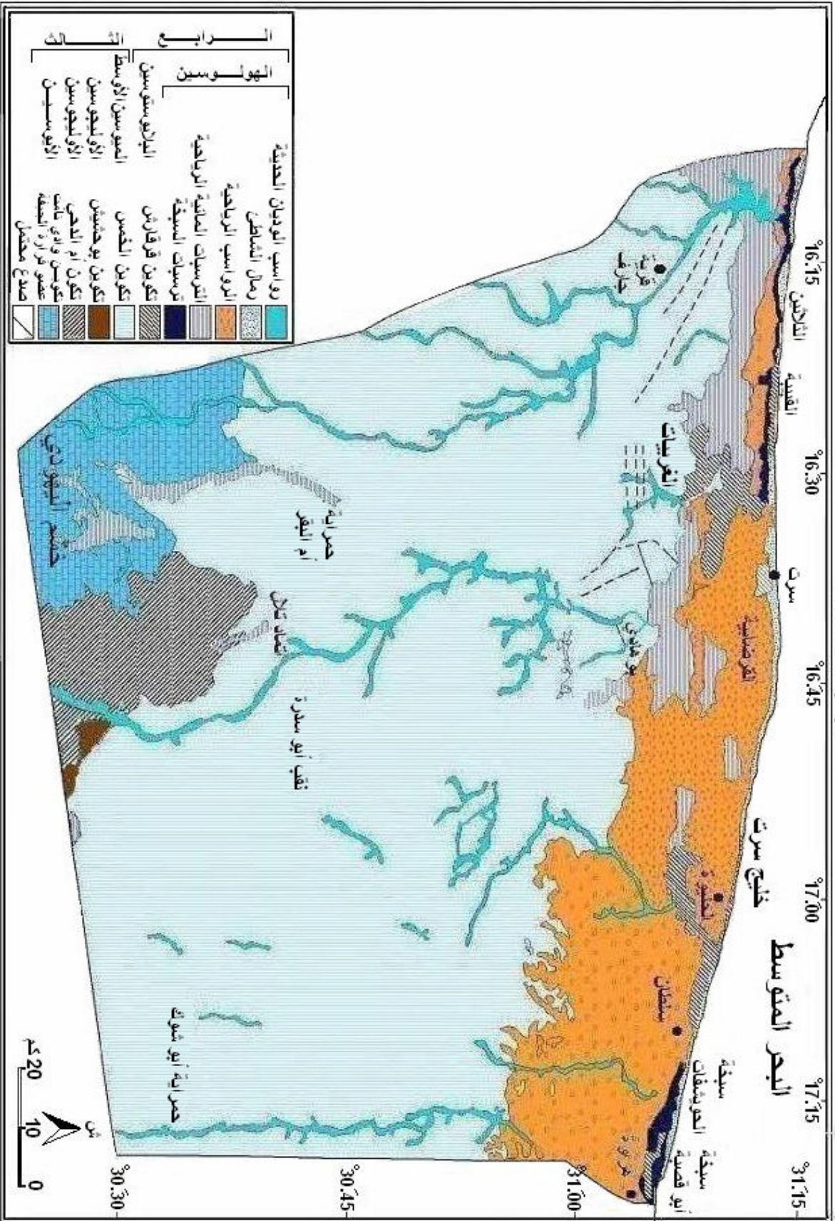
شكل رقم (2) جيولوجية منطقة الدراسة
